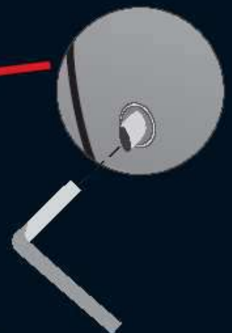
DETALLE A Sistema de fijación de tubos con tornillo cilíndrico con hexágono interior "Allen"
